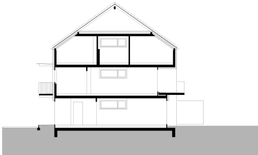
SCHNITT Bauteil 2
