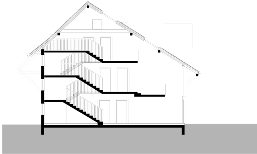
SCHNITT Bauteil 1
